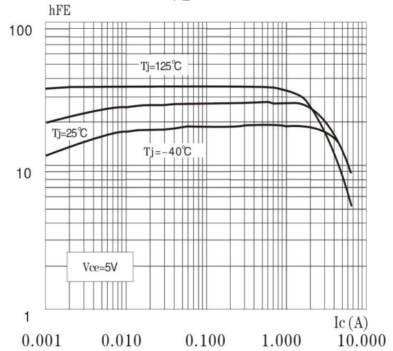
h_{FE} - I_c
